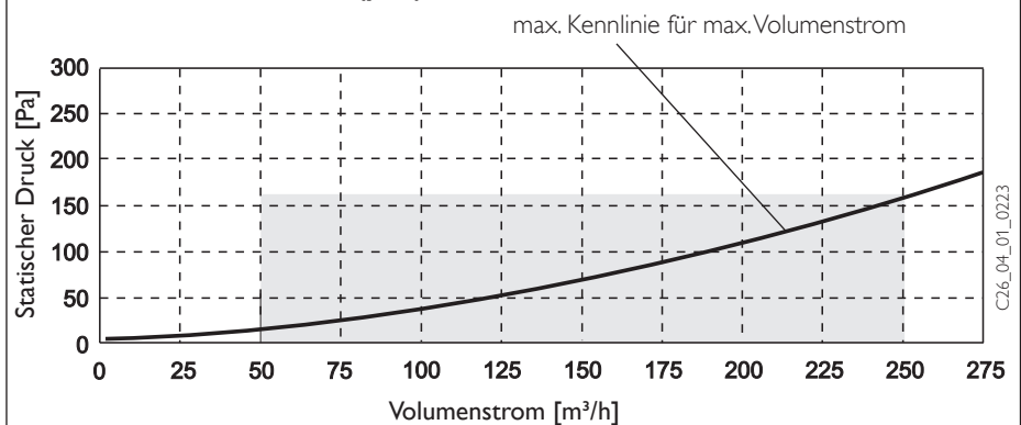
Lüfter-Kennlinie LWZ 170 (plus)
