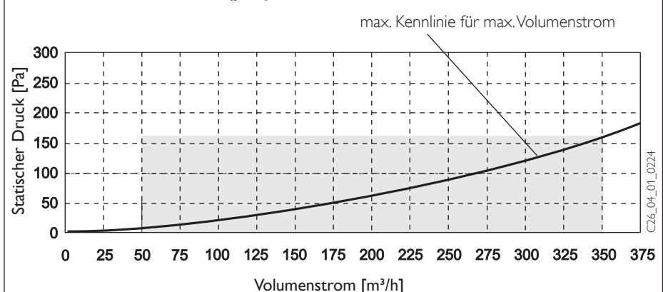
Lüfter-Kennlinie LWZ 270 (plus)
